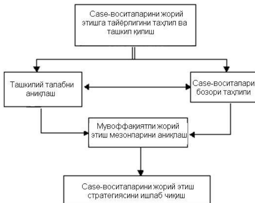
6.3.1-rasm. CASE-vositalariga bo'lgan talablar.
