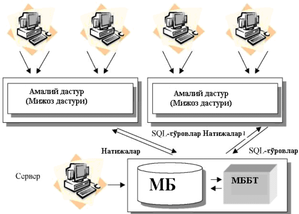
7.1.3-rasm. 'Mijoz-server' arxitekturasi
