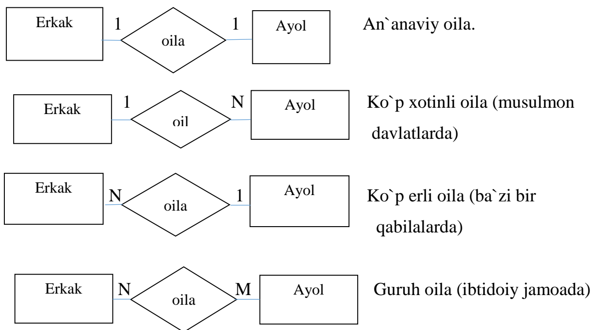
2.4.1-rasm. Ayol va erkak mohiyatlarining bog'lanishi
