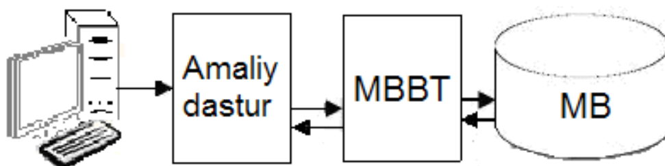
7.1.1-rasm. Markazlashgan arxitektura
