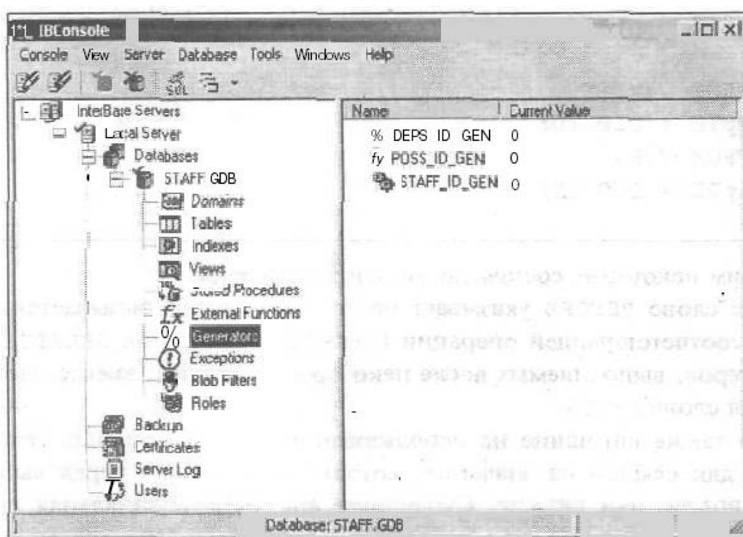
9.6.5-rasm. IBConsole dastur oynasida “Generators” ob’yektlarining ko’rinishi
