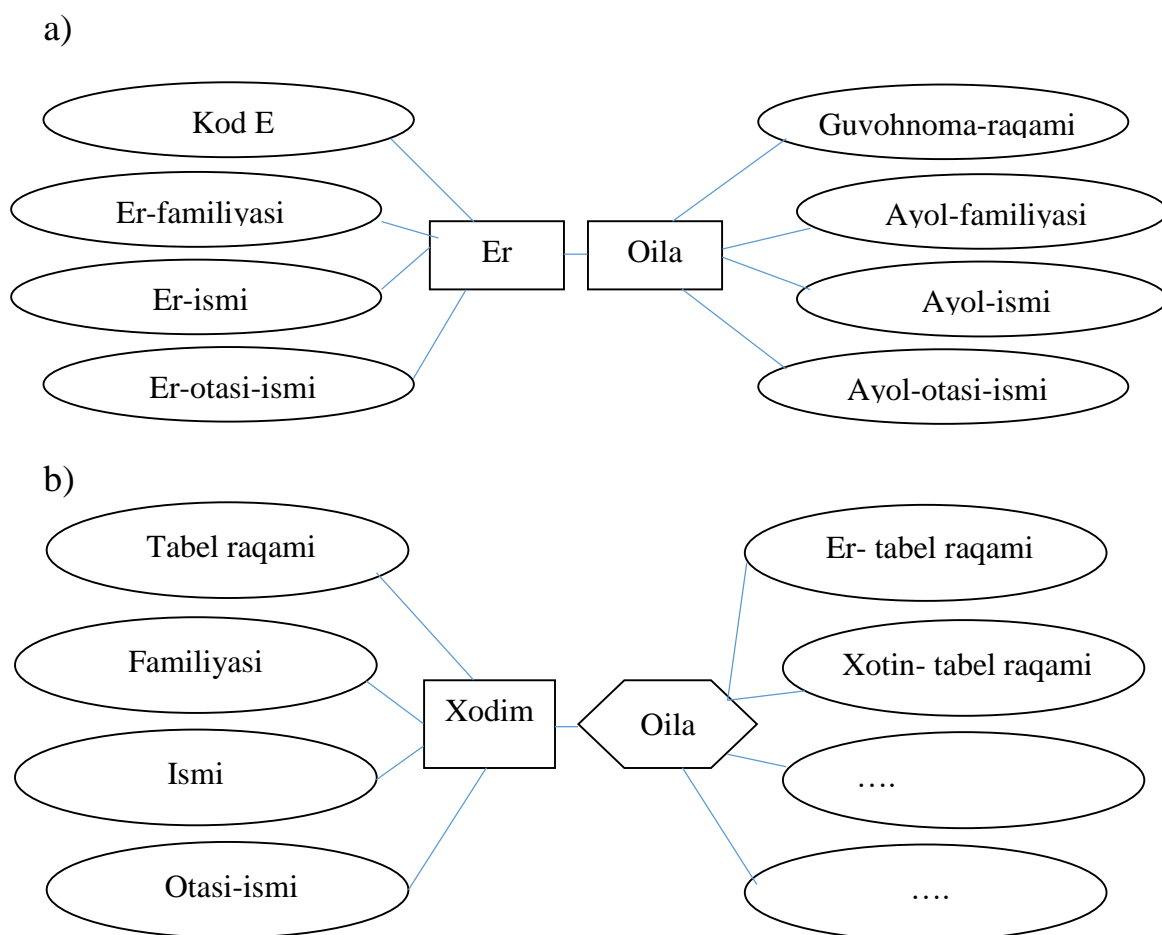
2.4.6-rasm. a) Oila va b) xodim mohiyatlari uchun ER diagramma
