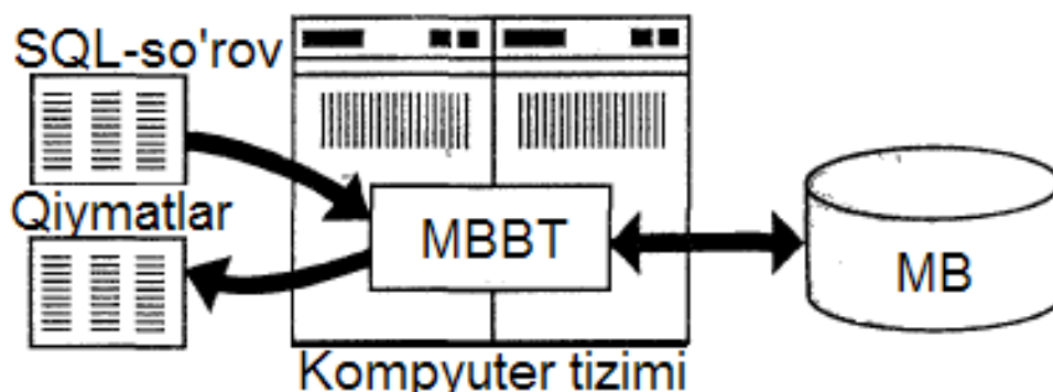
8.6.1-rasm. SQL so`rovni uzatish mexanizmi
