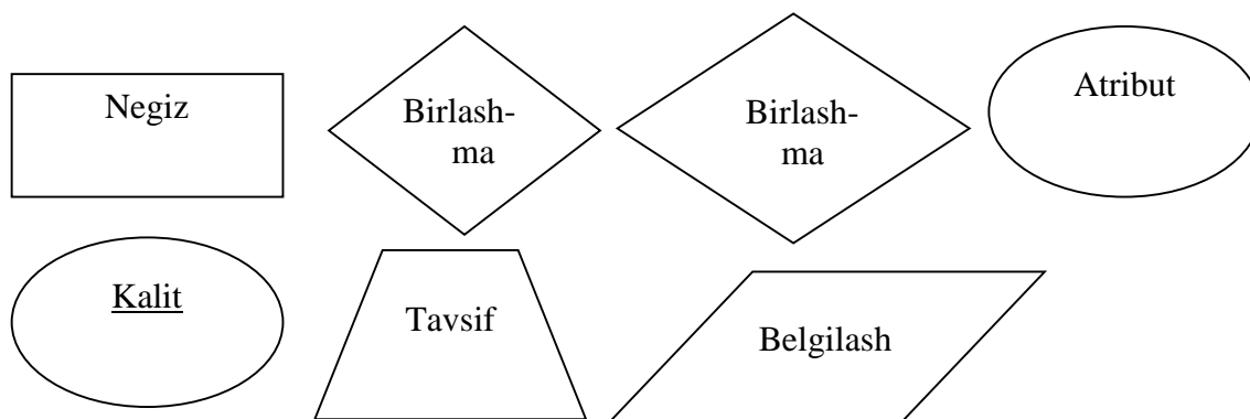
2.4.7-rasm. Kengaytirilgan ER diagramma tili elementlari
