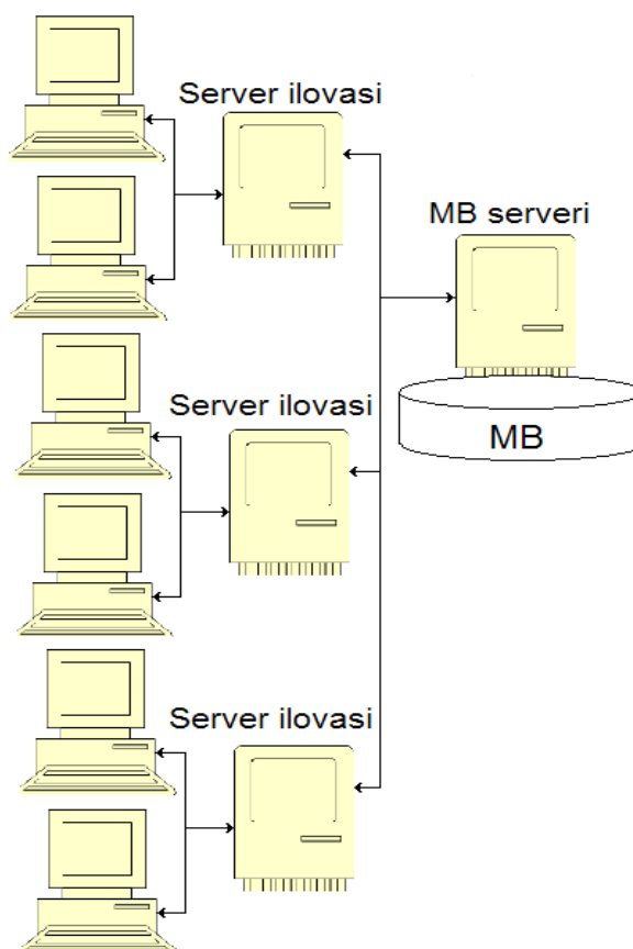
7.1.4-rasm. Uch zvenoli arxitektura
