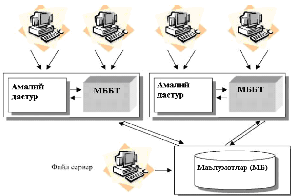
7.1.2-rasm. ‘Fayl-server’ arxitekturasi
