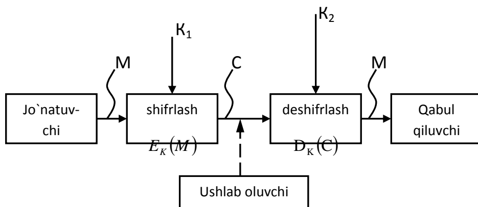
21.2-rasm. Ochiq kalitli asimmetrik kriptotizimning umumlashma sxemasi.
