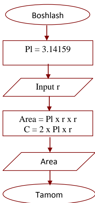
11.2-rasm. R radiusga ega aylananing uzinasi va yuzini topish blok chizmasi.
