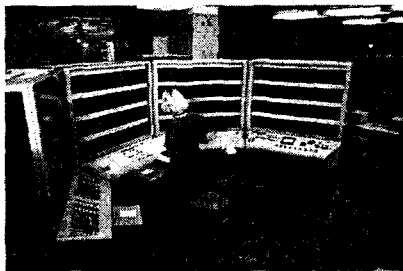
1.10-rasm. BESM-6.
