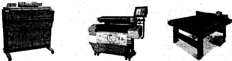
2.34-rasm. Plotterlar.
