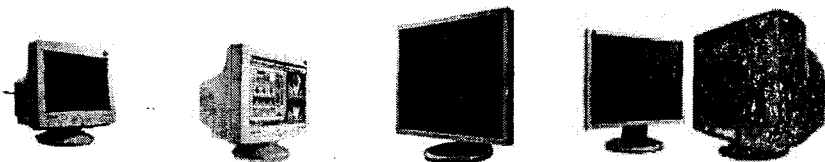
2.17-rasm. Monitorlar.
