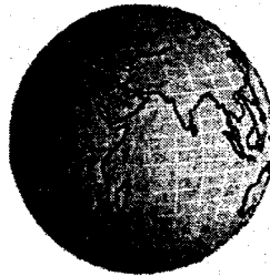
World
