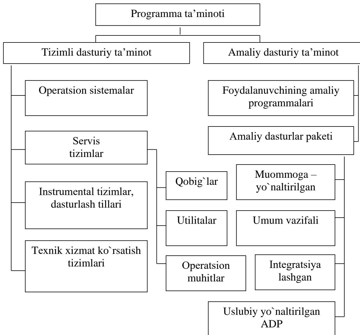
9.1-rasm. Dasturiy ta`minot tarkibi
