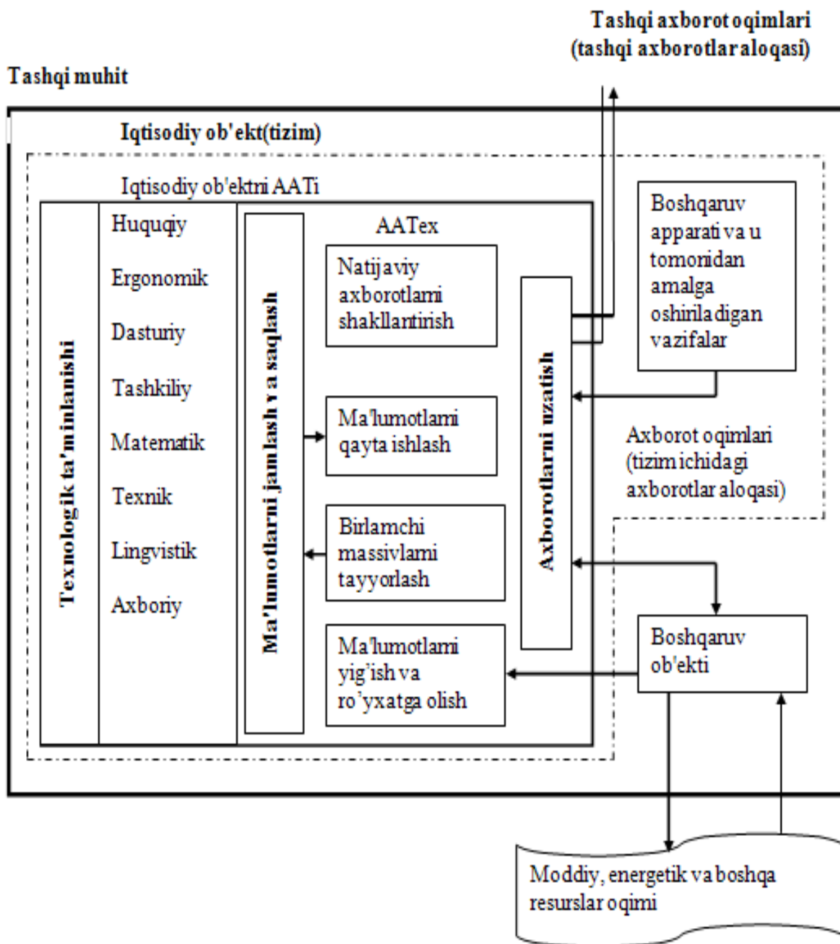
10.1- rasm. AAT va AATexning tuzilishi
