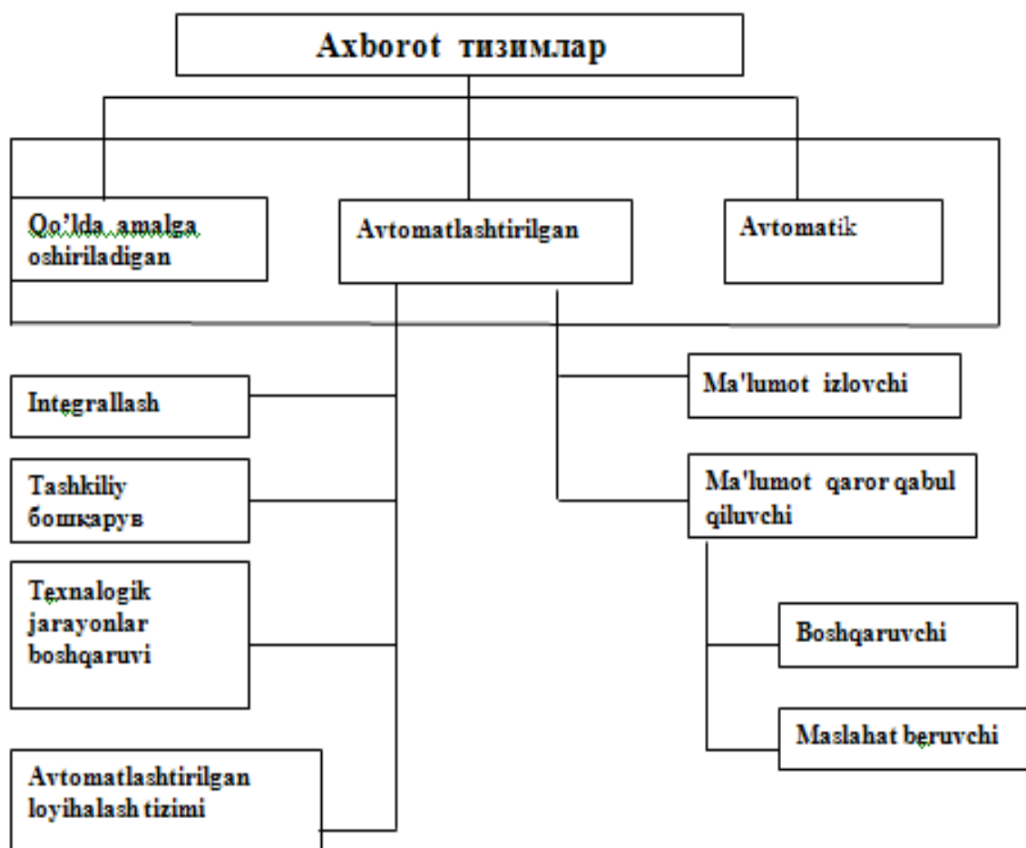
3.14-rasm. Har xil alomatga ko`ra AT klassifikatsiyasi 17
