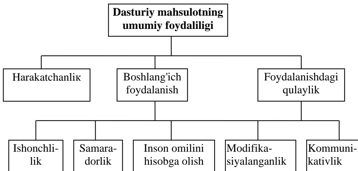
9.2.-rasm. Dasturiy mahsulotlarning sifat xususiyatlari
