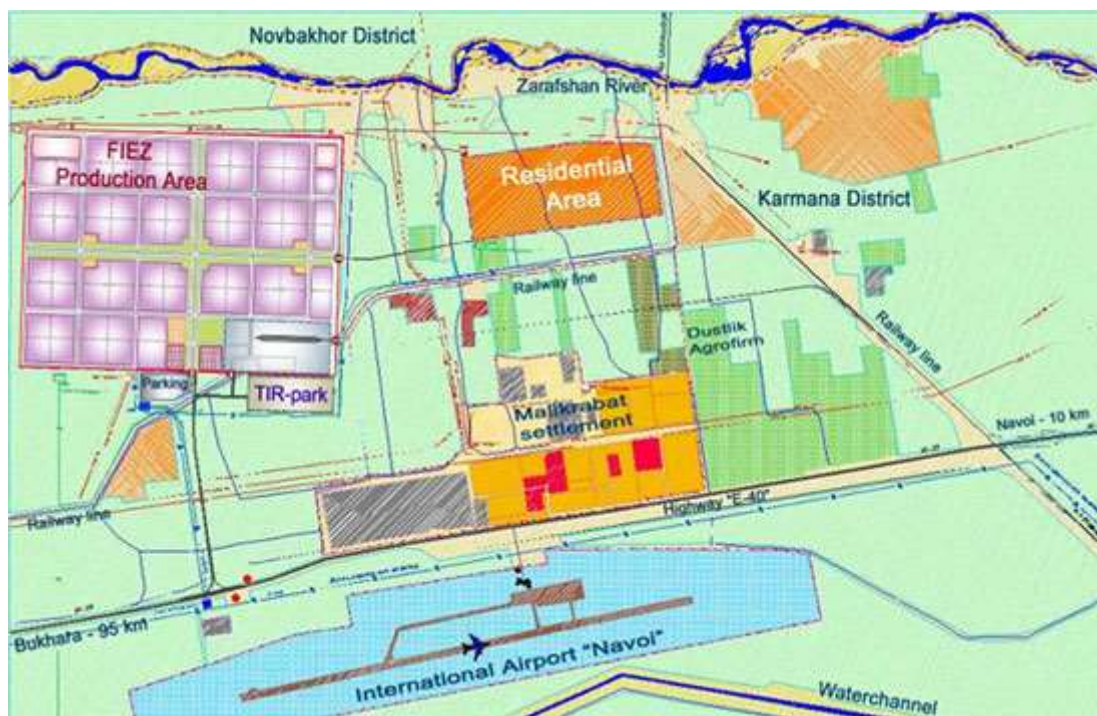
7.10-расм. “Навоий” эркин индустриал-иқтисодий ҳудудининг мултимодал транспорт логистика узели *
