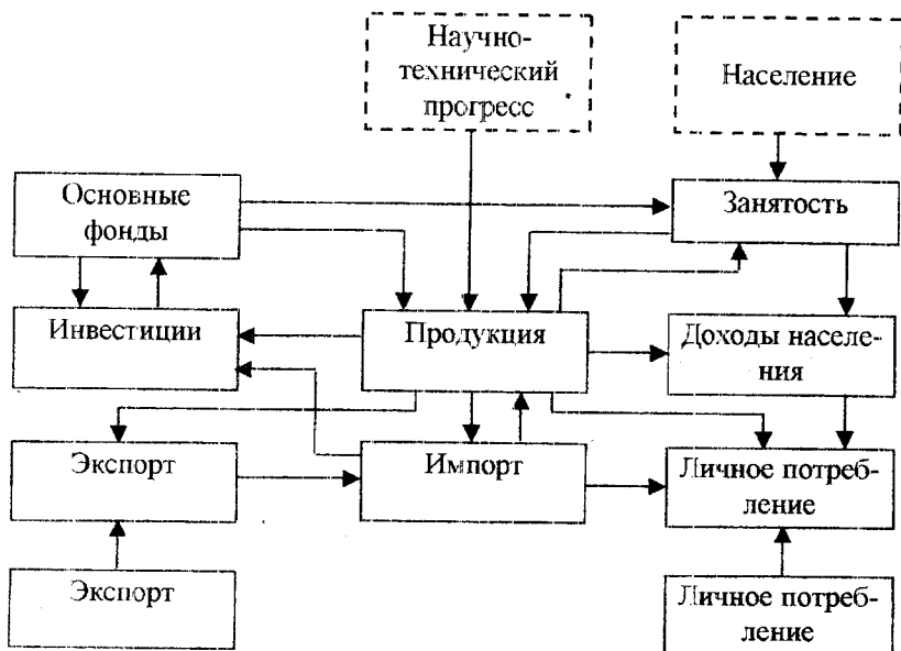
Рис. 5.2 Основные блоки переменных и их связи в комплексной эконометрической модели
