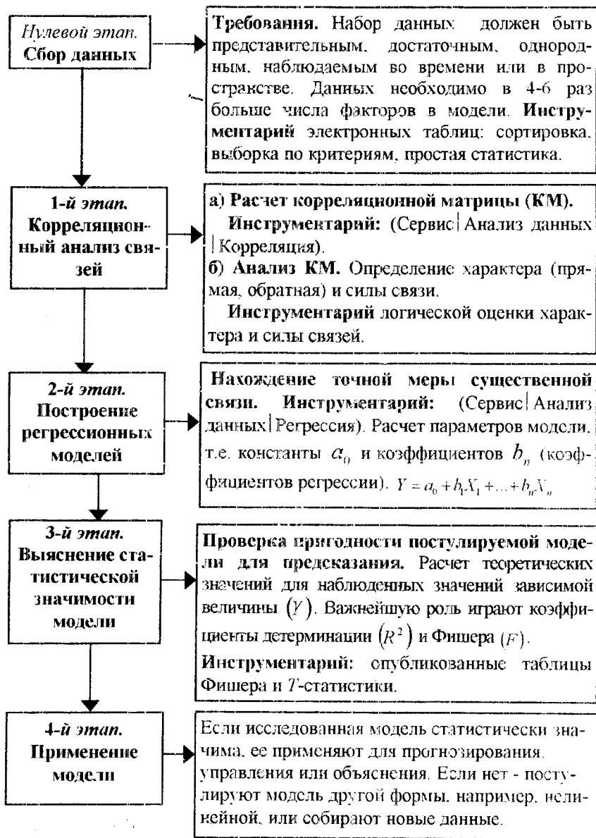
Рис.13.1. Этапы корреляционно-регрессионного анализа.
