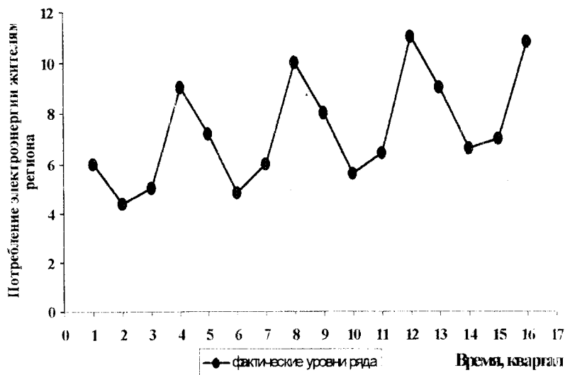
Рис. 1.3. Потребление электроэнергии жителями региона
