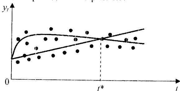
Рис. 1.5. Ошибка спецификации при выборе уравнения тренда
