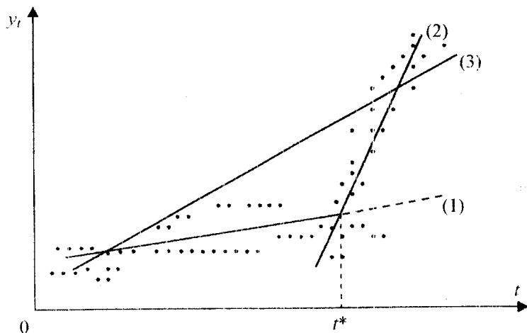
Рис. 1.6. Изменение характера тенденции временного ряда
