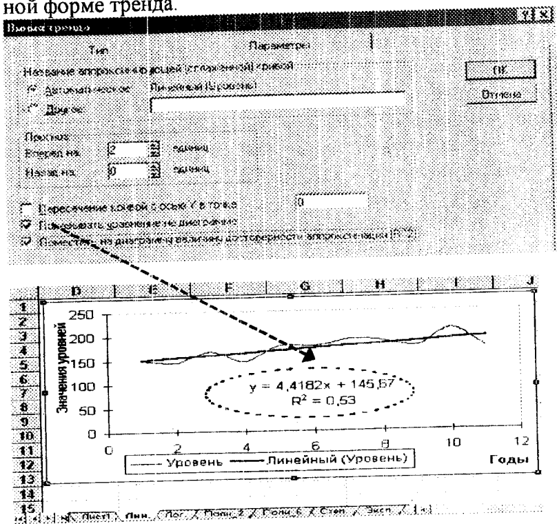
Рис. 13.12. Вверху: настройка параметров тренда. Настроен вывод уравнения на диаграмму и вывод R^2 . Внизу: результат настройки, полученный после активизации кнопки ОК.
