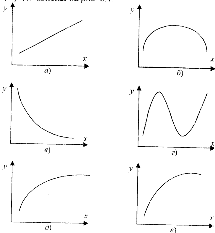
Рис. 8.1. Основные типы кривых, используемые при количественной оценке связей между двумя переменными:
