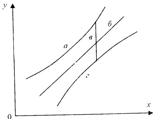
Рис. 8.4. Доверительный интервал линии регрессии:
