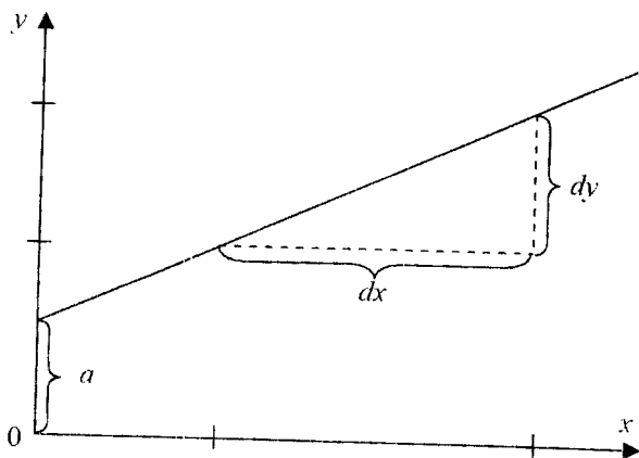
Рис. 8.2. Графическая оценка параметров линейной регрессии
