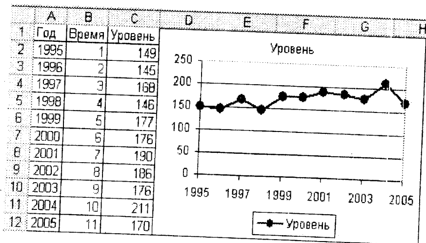
Рис. 13.11. Диаграмма исходного динамического ряда (вверху) и диаграмма преобразованного (ниже). Для нормальной работы вычислительных программ моделирования трендов в Excel многозначные периоды следует заменить их номерами (с учетом расстояния между позициями).
