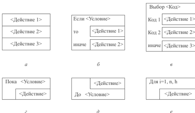
Рис. 2.7. Условные обозначения Flow-форм для основных конструкций: a – следование; б – ветвление; в – выбор; г – цикл-пока; д – цикл-до; е – счетный цикл
