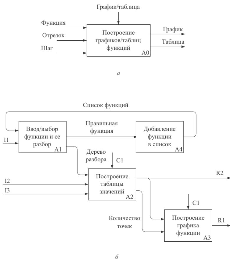
Рис. 4.10. Функциональные диаграммы для системы исследования функций:
