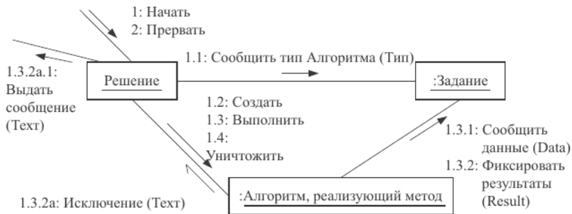
Рис. 7.10. Диаграмма кооперации сценария Процесс решения
