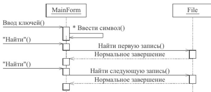
Рис. 9.13. Диаграммы последовательностей действий: a – запуск приложения; б – добавление записей; в – поиск записей
