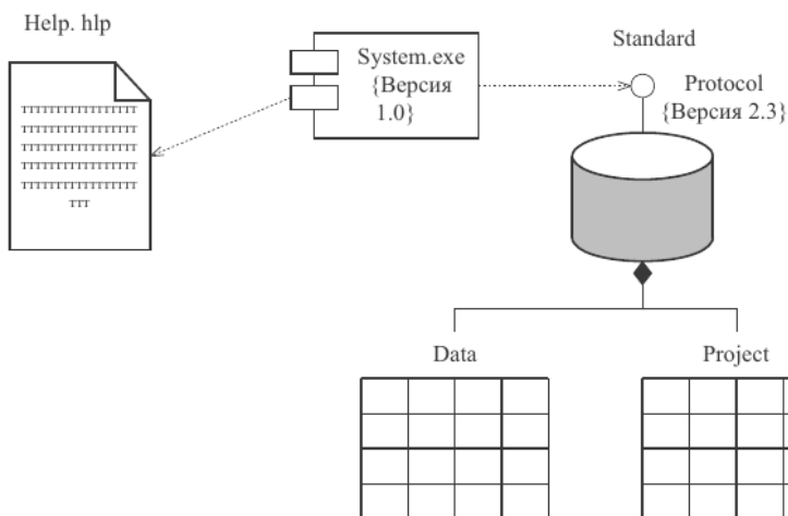
Рис. 7.24. Диаграмма компонентов системы решения комбинаторно-оптимизационных задач с указанием интерфейса
