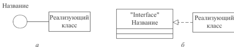
Рис. 7.14. Условные обозначения реализации интерфейсов:
