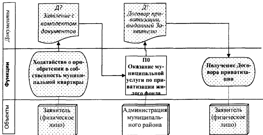
Рис. 2.39. Пример диаграммы BFSH с учетом УФО-подхода. Контекст
