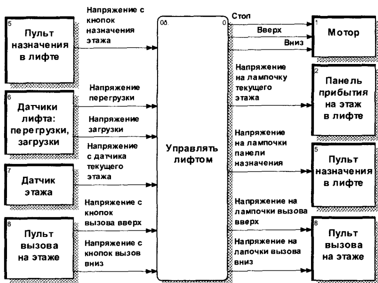
Рис. 3.1. Контекстная DFD-диаграмма ECS
