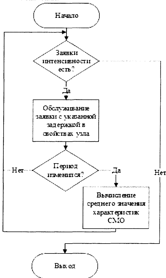
Рис. 3.94. Алгоритм узла «Обработка» одноканальной СМО с отказами
