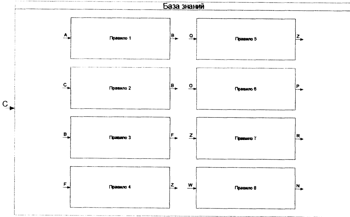
Рис. 2.48. База продукционных правил в терминах УФО-подхода
