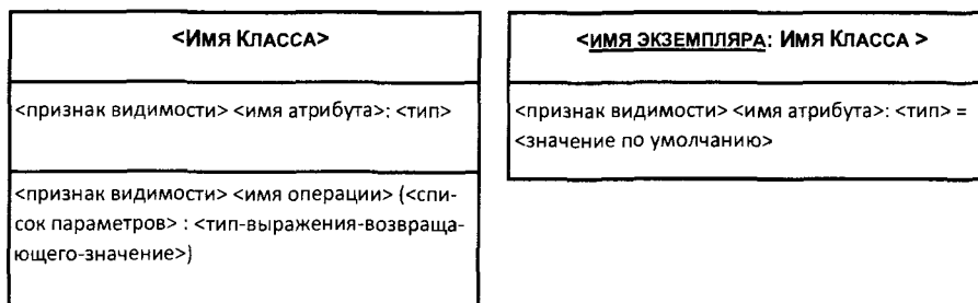
Рис. 3.20. Графическое изображение класса и экземпляра
