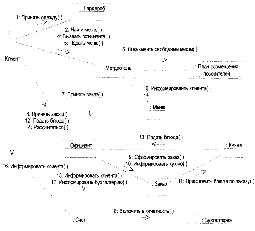
Рис. 3.34. О-модель (внутренняя модель) бизнес-системы «Ресторан». Диаграмма кооперации объектов для прецедента «Обслуживание обеда/ужина»
