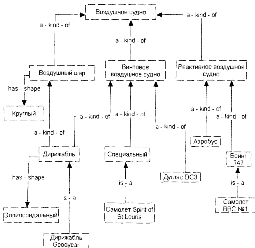
Рис. 2.58. Модель понятий и отношений между ними в терминах COMПЗ
