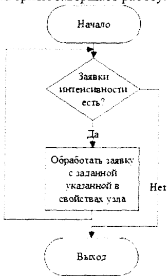
Рис. 3.105 Алгоритм узлов «Обработка», «Обработка2», «Обработка3» многоканальной СМО с ограниченной длиной очереди
