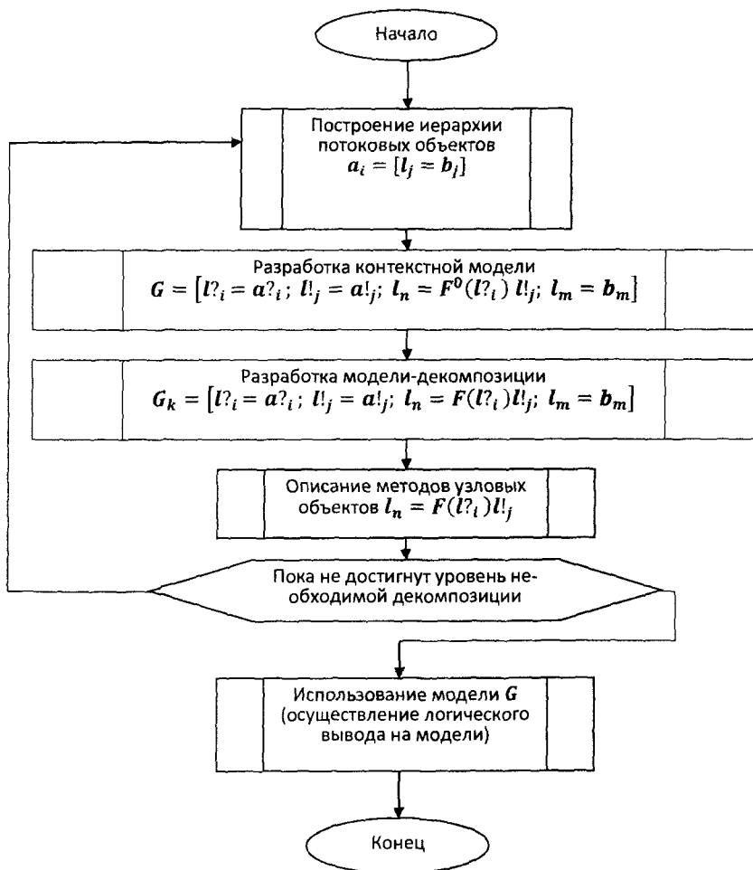
Рис. 2.64. Алгоритм описания знаний с помощью COMPT
