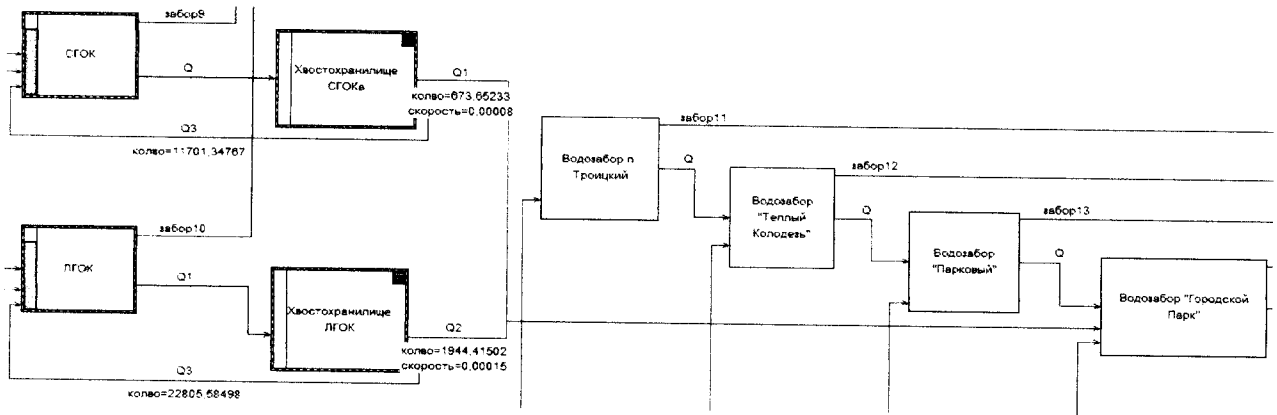
Рис. 3.83. Очистка и транспортировка воды из хвостохранилищ в ГОКи
