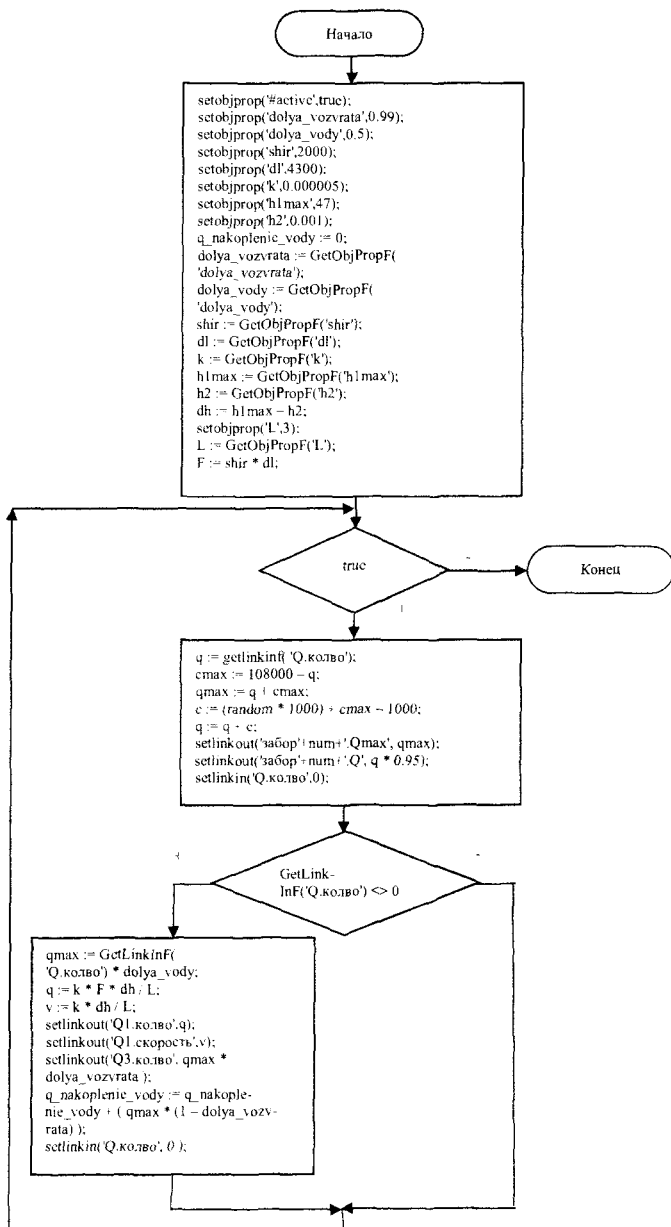
Рис. 1. Алгоритм метода узлового объекта «Хвостохранилище СГОКа» в терминах языка описания функциональных объектов
