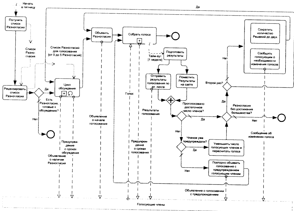
Рис. 3.38. Пример диаграммы в нотации BPMN. Голосование по электронной почте
