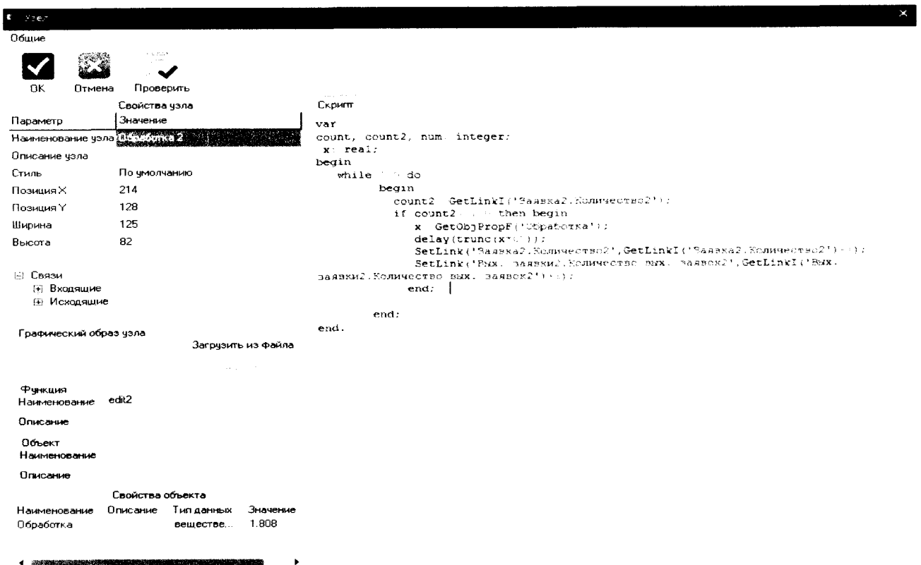
Рис. 3.107. Фрагмент кода узла «Обработка 2» многоканальной СМО с ограниченной длиной очереди
