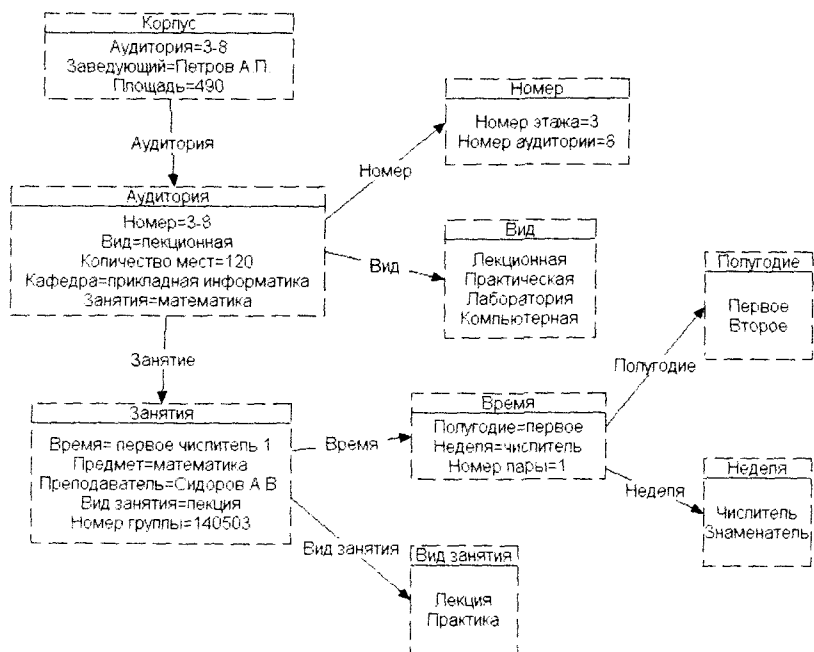
Рис. 2.60. Результат применения операции префиксного действия к фреймовой сети средствами СОМПЗ
