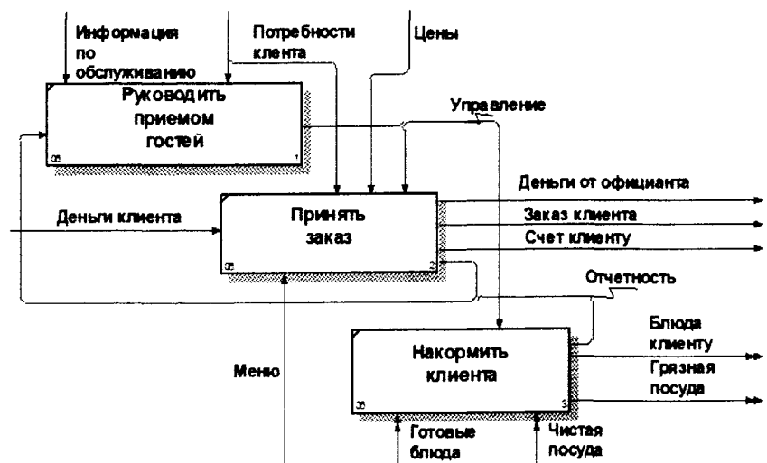
Рис. 3.15. SADT-диаграмма ресторана второго уровня (обслуживание клиентов)
