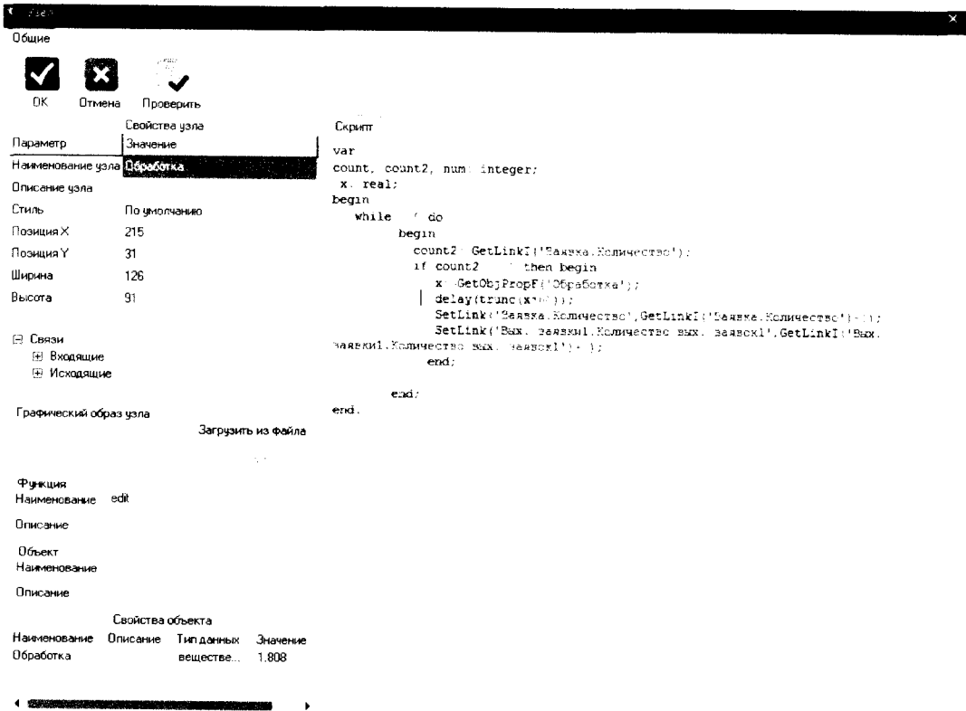
Рис. 3.106. Фрагмент кода узла «Обработка» многоканальной СМО с ограниченной длиной очереди
