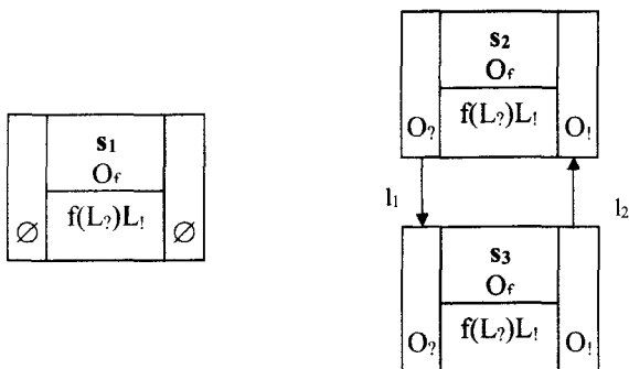
Рис. 2.34. Модель до оптимизации по принципу коммуникативности
