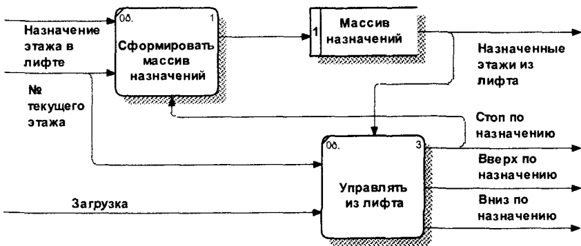
Рис. 3.4. DFD-диаграмма третьего уровня (обработка назначений)
