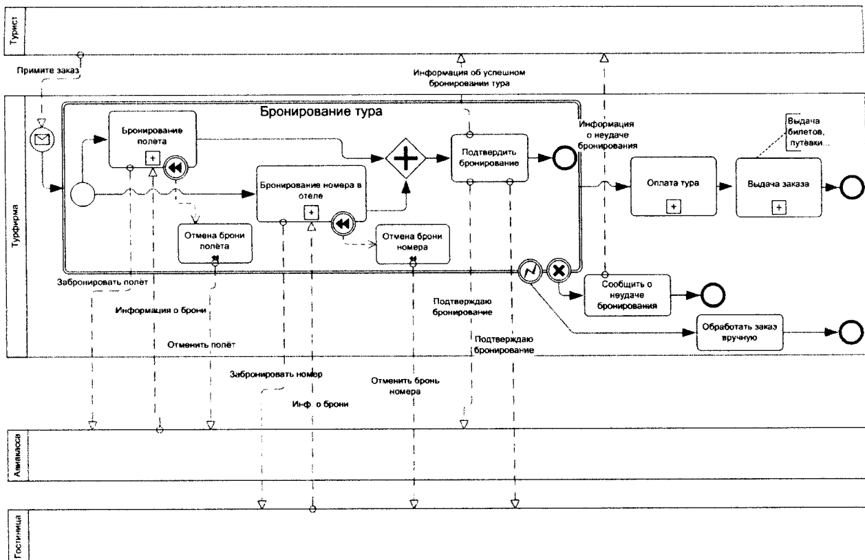
Рис. 3.39. Пример диаграммы в нотации BPMN. Деятельность турфирмы
