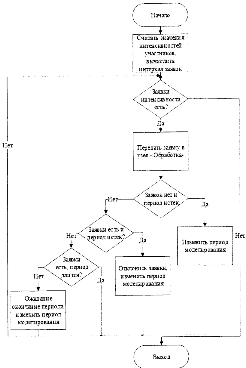
рис. 4.11 Алгоритм функционирования узла «Клиенты» одноканальной СМО с отказами
