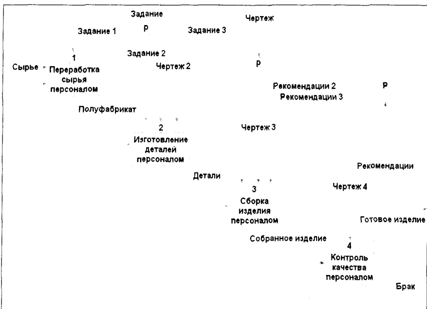
Рис. 3.61. Диаграмма декомпозиции на рис.3.11 в виде модели «Узел-Функция-Объект»
