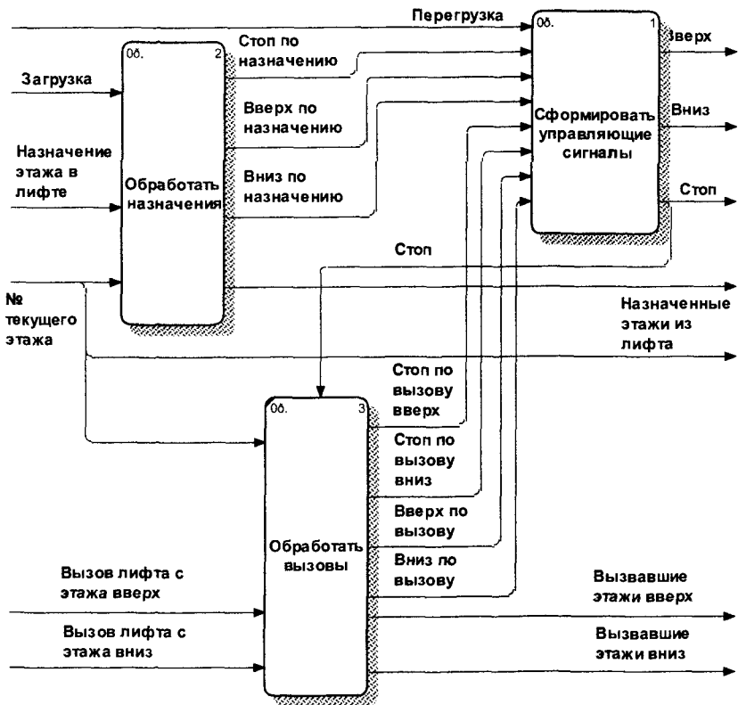
Рис. 3.3. DFD-диаграмма второго уровня (процесс принятия решений)
