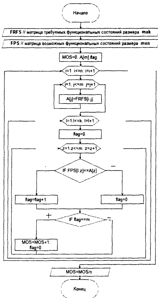
Рис. 2.23. Алгоритм расчета меры системности
