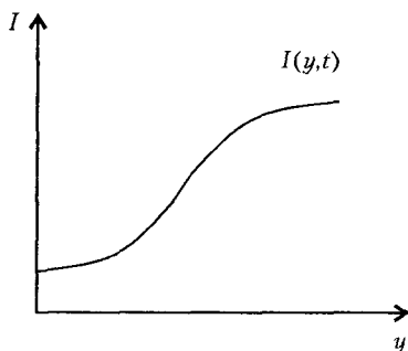
Рис. 9.10. Функция инвестиций Калдора
