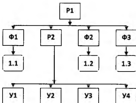
Чизиқли функционал
