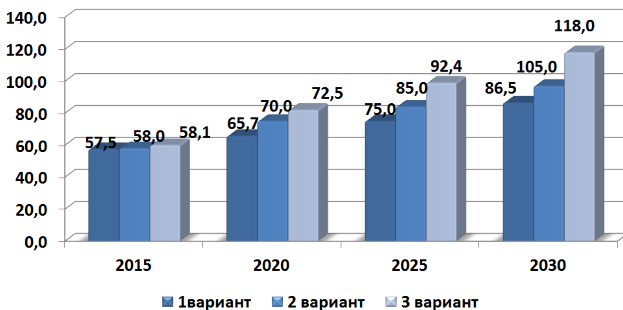
Рисунок 3. Динамика и прогноз спроса на электроэнергию 21
