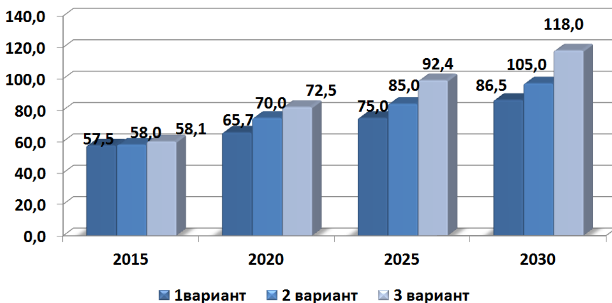
3-расм. Электр энергияга талабни прогнозлаш ва баҳолаш динамикаси 21
