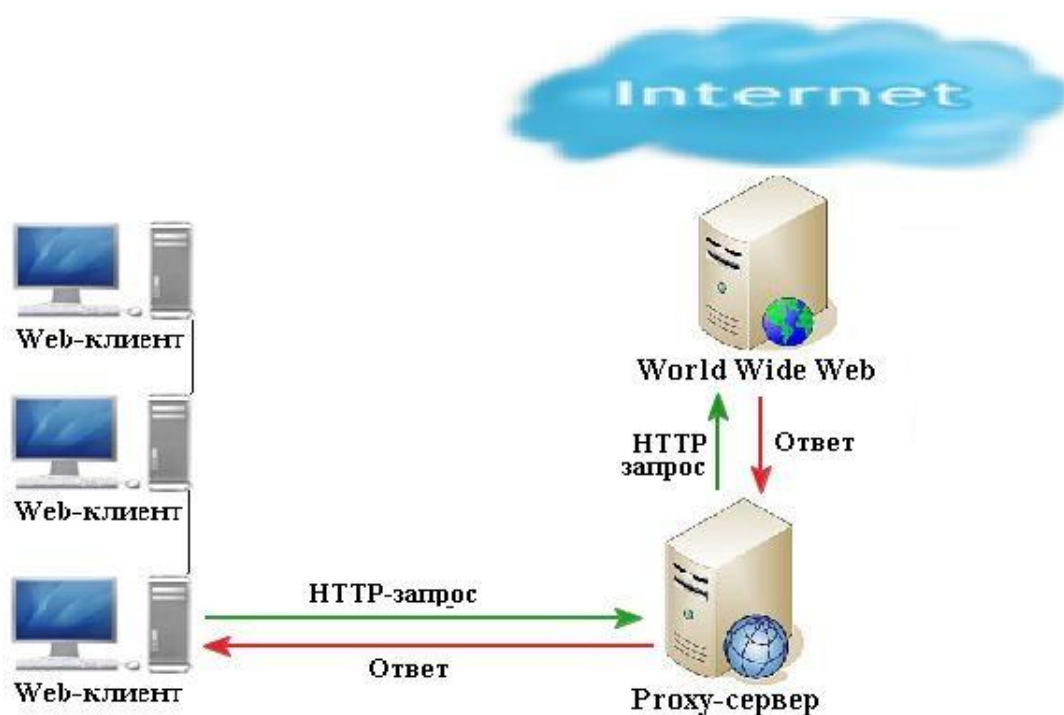
Рис. 21.6. Пример установления соединения с веб-сервером через прокси-сервер 170
