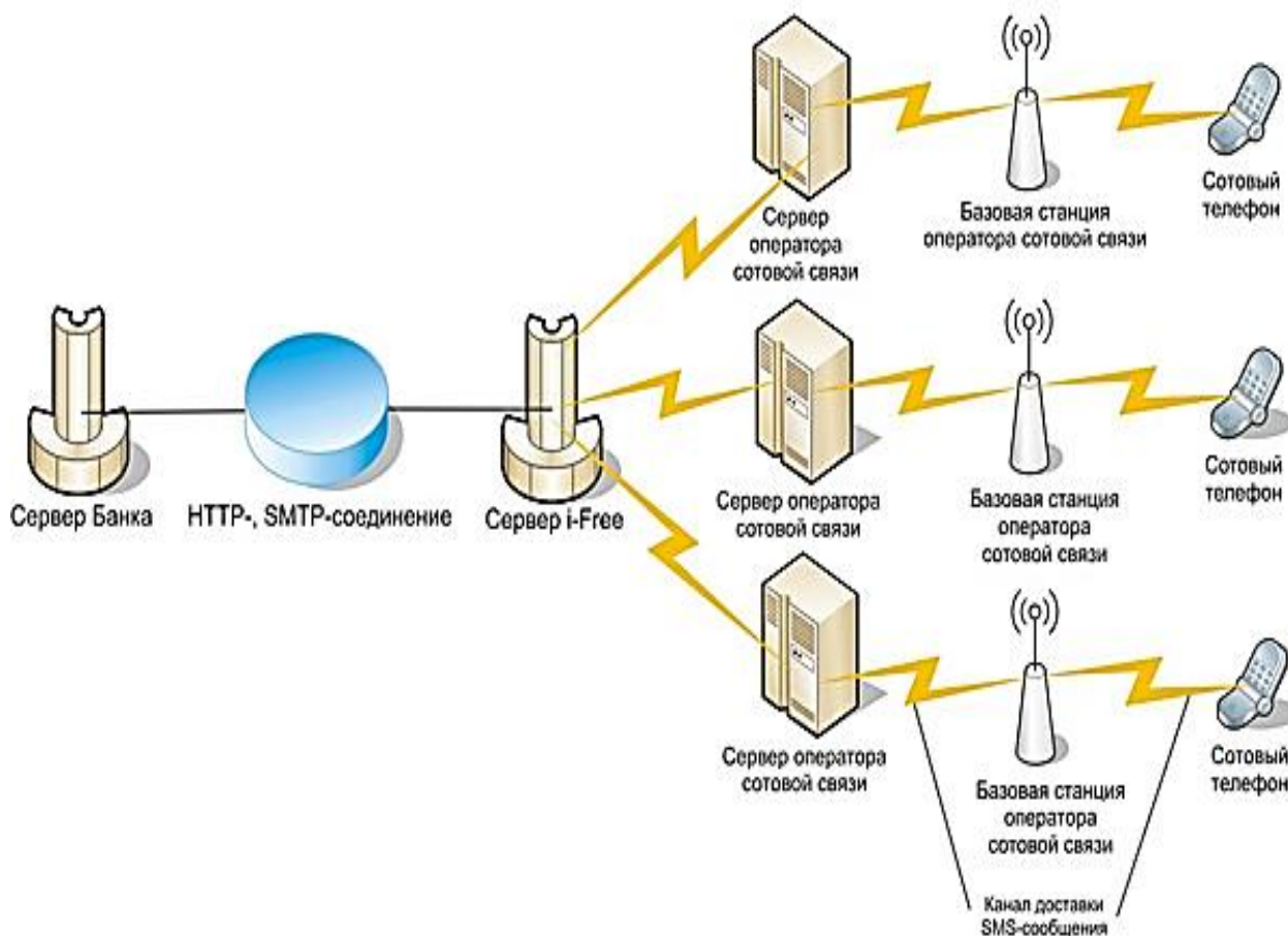
Рис. 18.19. Схема соединения сервера банка с сервером провайдера 132
