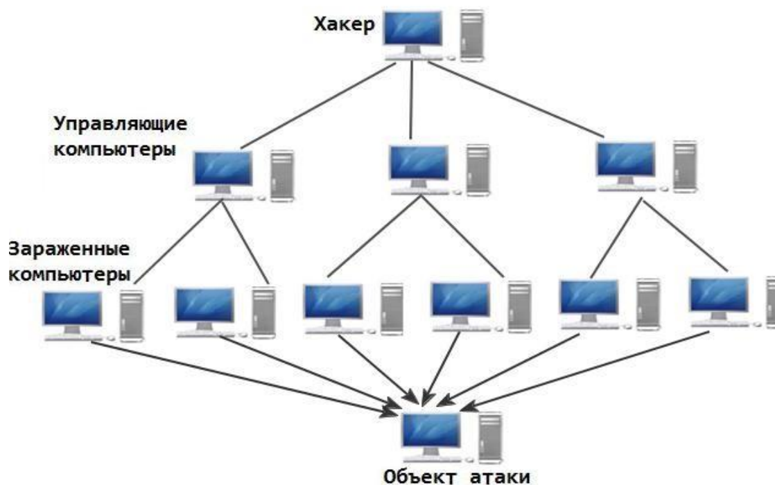
Рис. 21.4. Принцип действия DDoS-атак 168
