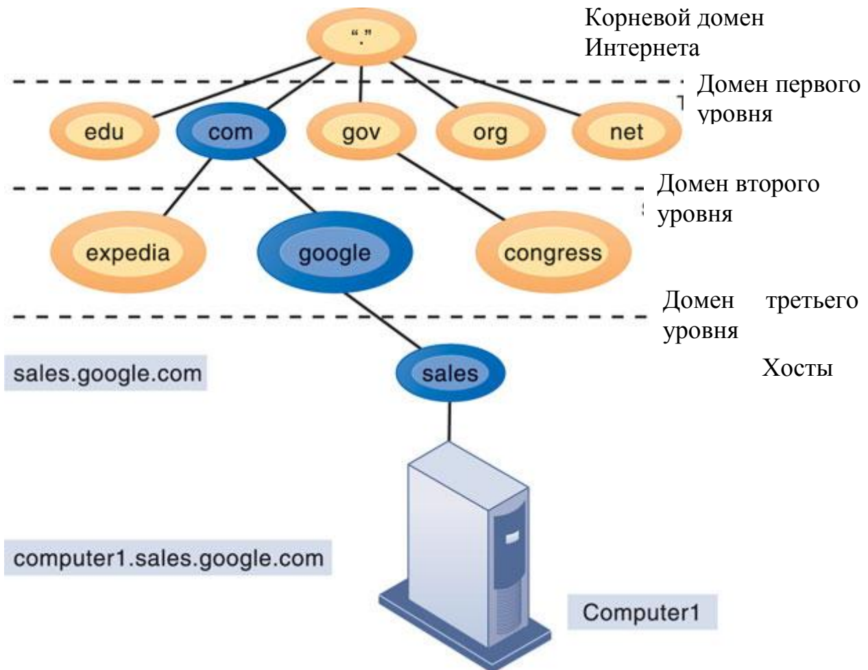
Рис. 9.9. Иерархия адресов интернета 42
