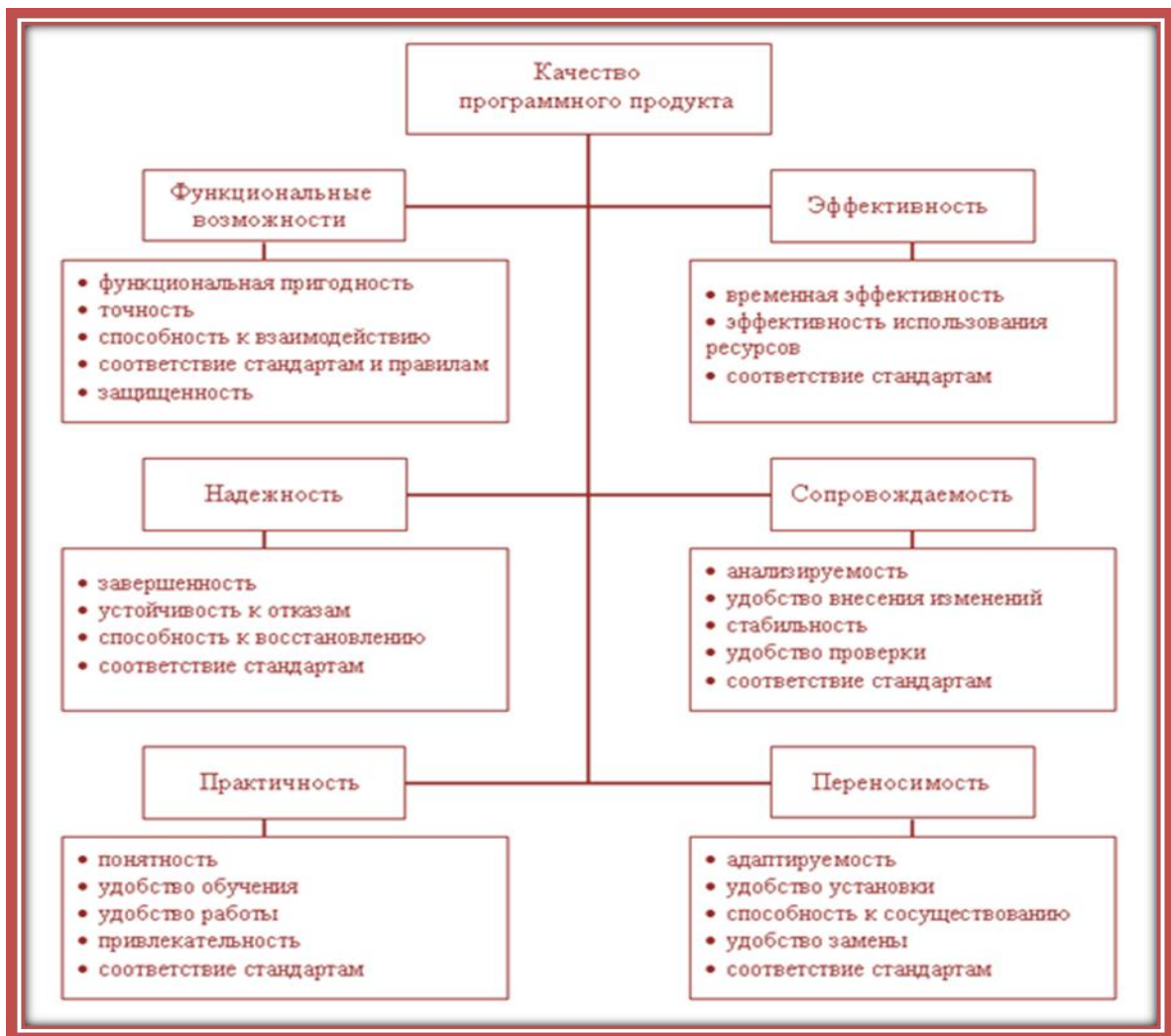
Рис. 10.5. Основные характеристики качества ПО 47
